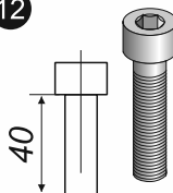
Винт М8х40(Возможна замена на болт с шестигранной головкой), 2 шт.
